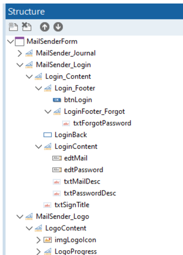
Рисунок 3.7 Загальний вигляд структури інтерфейсу в RadStudio
